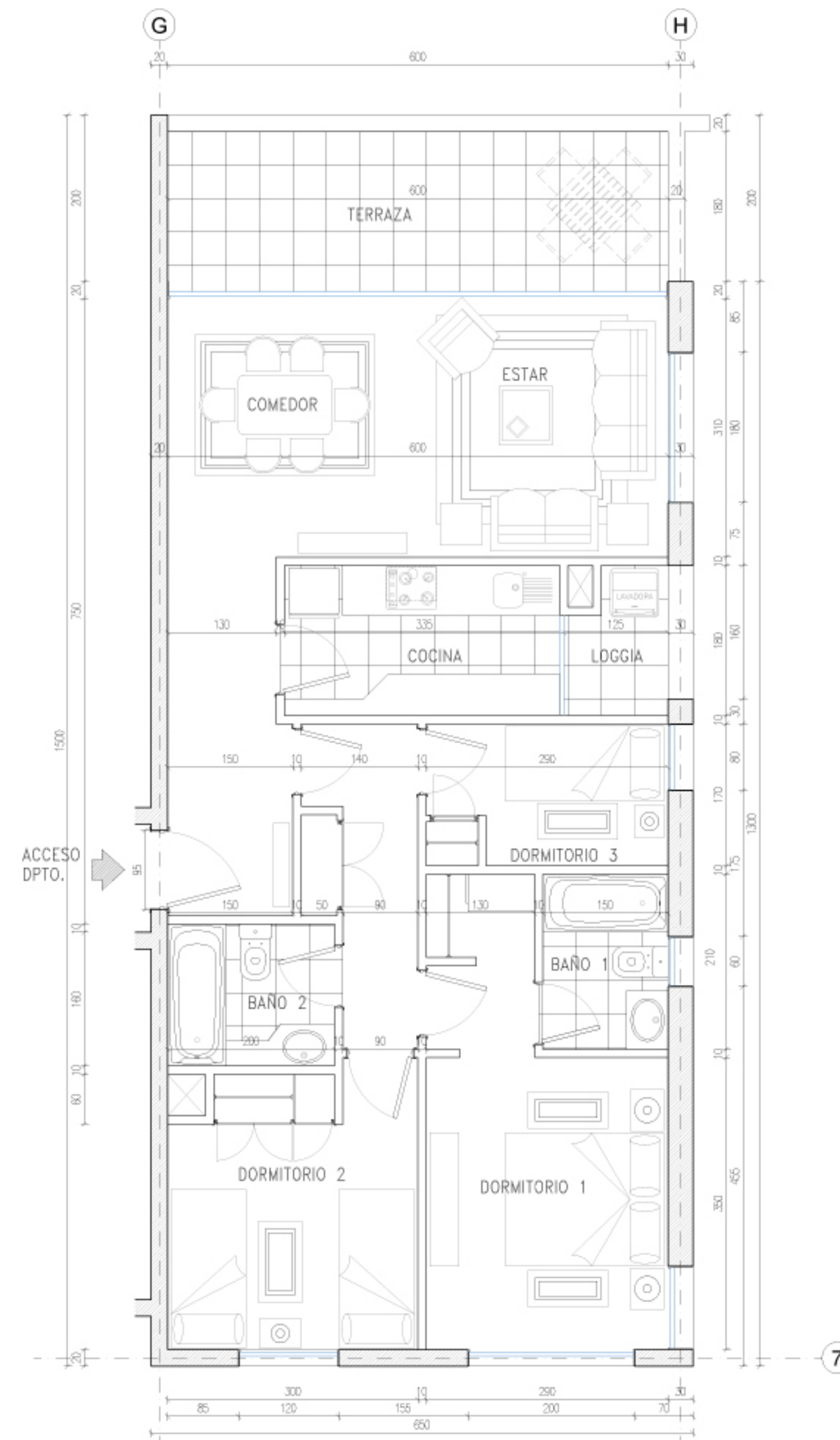
ALTERNATIVA 1 PLANTA TIPO DPTO.5 ESCALA 1:50
